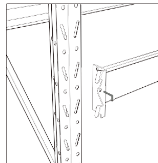
Рис 3. Установка балки на раму
